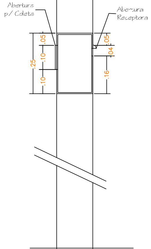
Corte X - X
